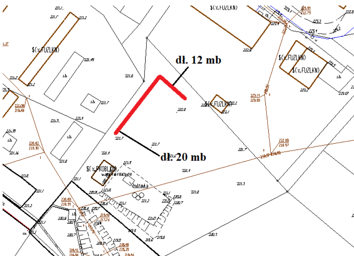
Rys. nr 1 Montaż i umiejscowienie piłkochwytu
