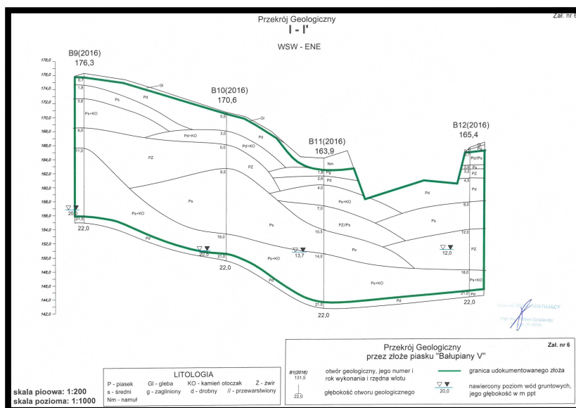
Rys. 25. Przekrój geologiczny przez udokumentowane złożo piasku „Bałupiany V”
