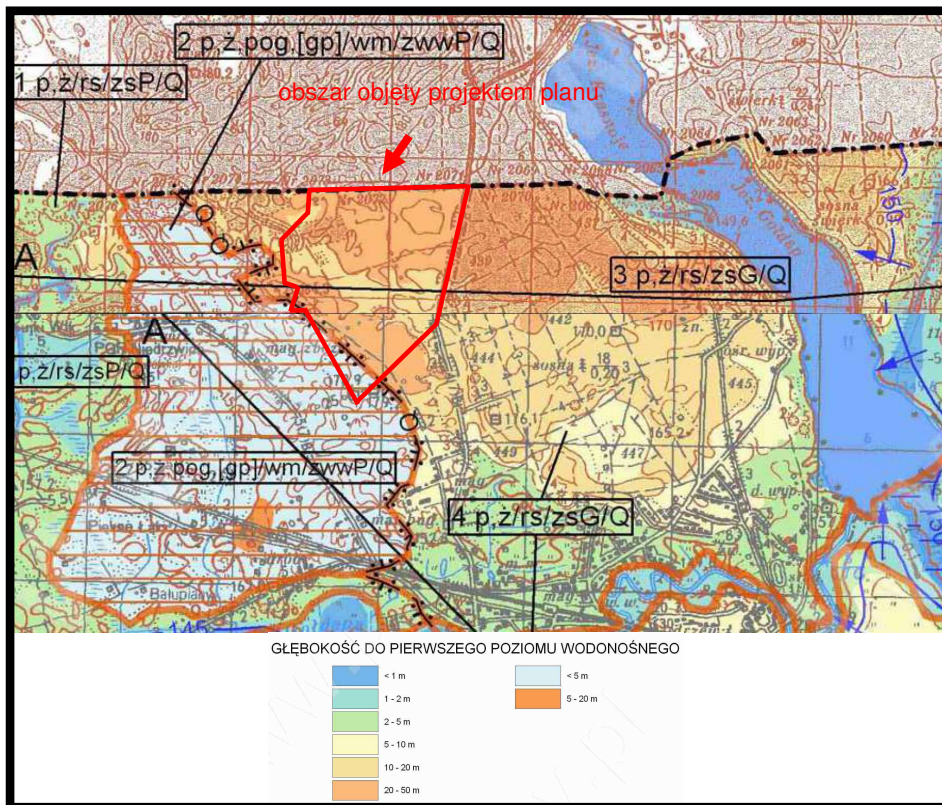
Rys. 18. Głębokość do pierwszego poziomu wodonośnego w rejonie obszaru objętego analizami – granice obszaru zaznaczono kolorem czerwonym
