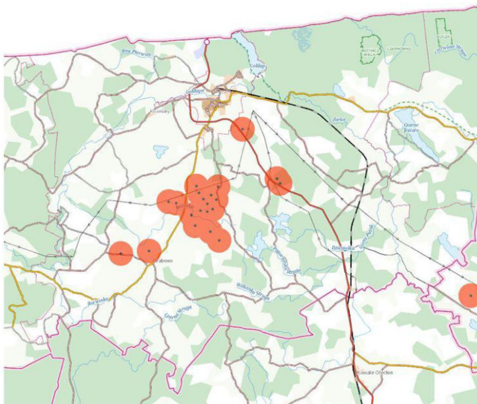
Ryc. 31 Lokalizacja wiatraków i stref wyłączonych z zabudowy mieszkaniowej na terenie gminy Gołdap
