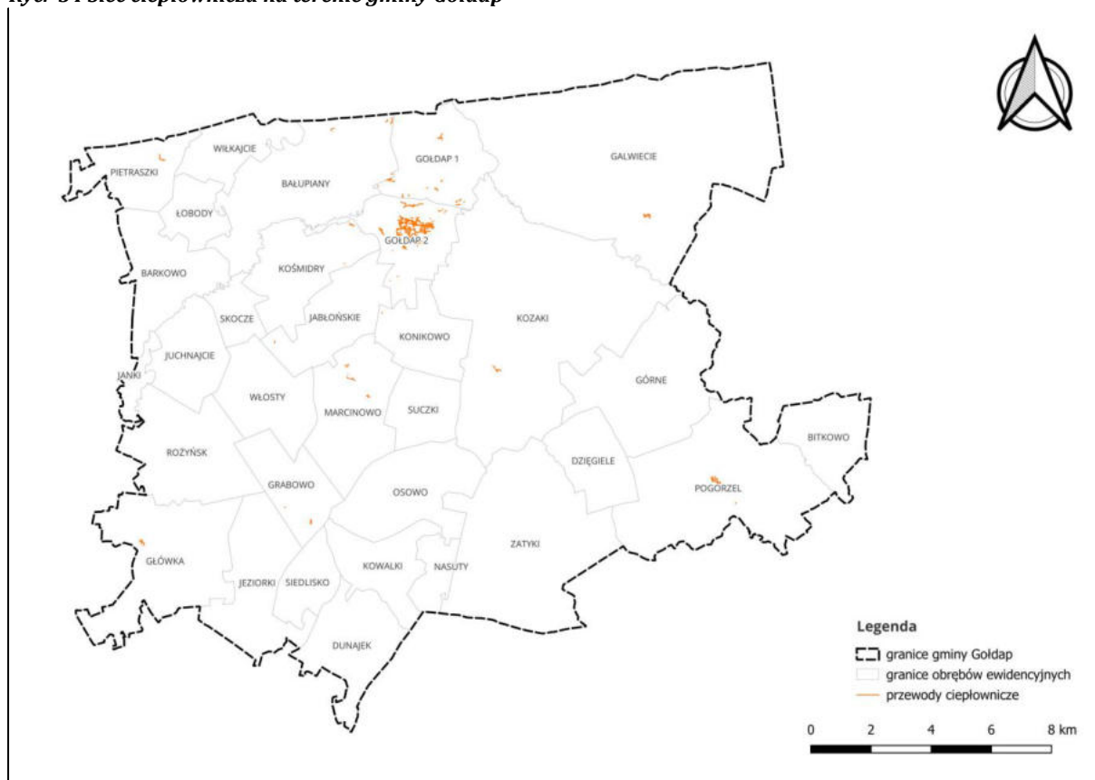
Ryc. 34 Sieć ciepłownicza na terenie gminy Gołdap
