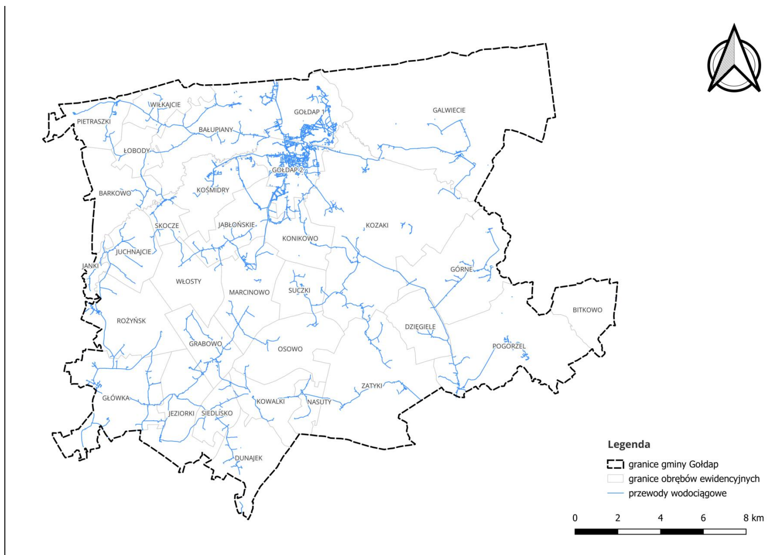
Ryc. 35 Sieć wodociągowa na terenie gminy Gołdap
