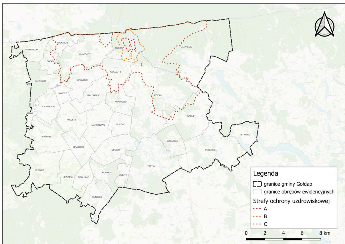
Ryc. 30 Granice stref ochronnych uzdrowiska Gołdap
