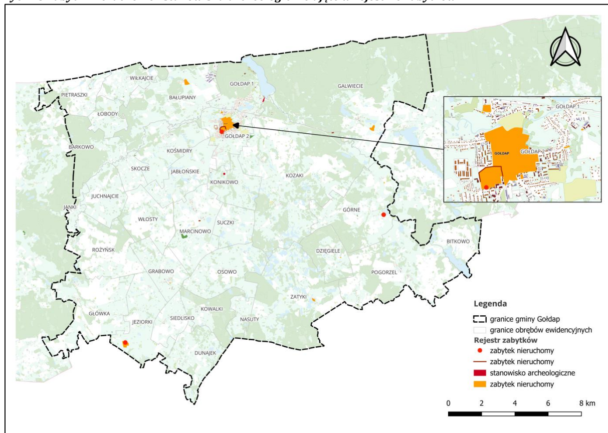
Ryc. 28 Zabytki nieruchome i stanowiska archeologiczne ujęte w rejestrze zabytków
