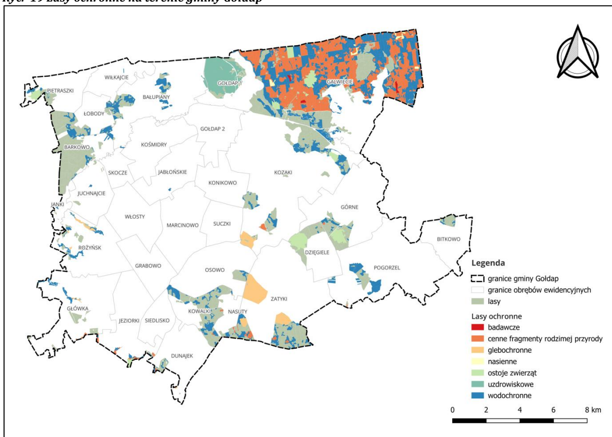
Ryc. 19 Lasy ochronne na terenie gminy Gołdap
