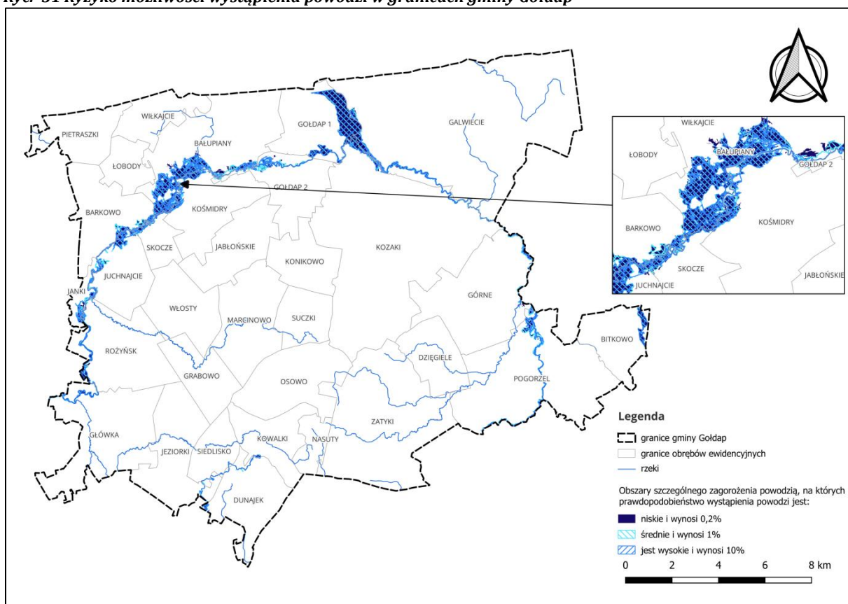
Ryc. 31 Ryzyko możliwości wystąpienia powodzi w granicach gminy Gołdap
