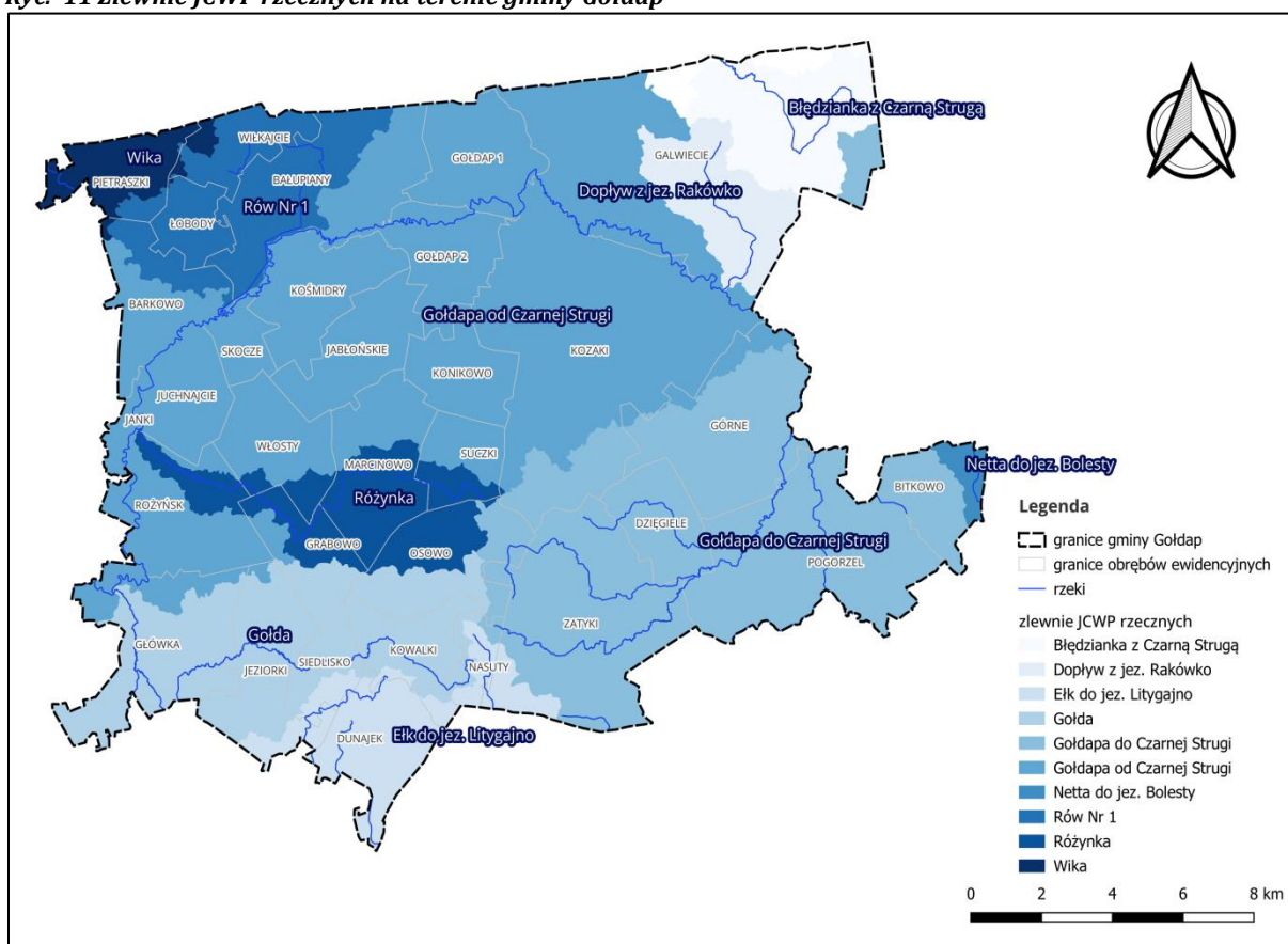
Ryc. 11 Zlewnie JCWP rzecznych na terenie gminy Gołdap
