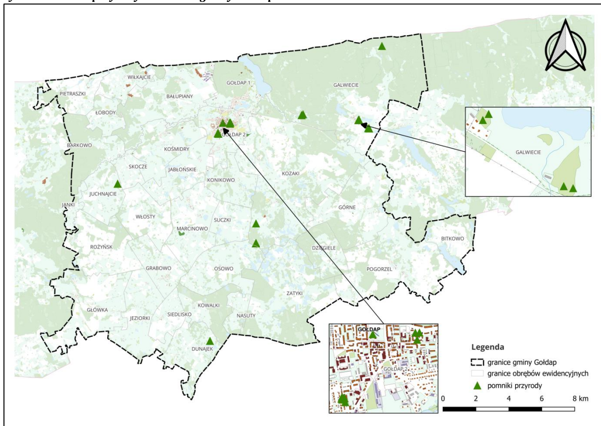
Ryc. 25 Pomniki przyrody na terenie gminy Gołdap
