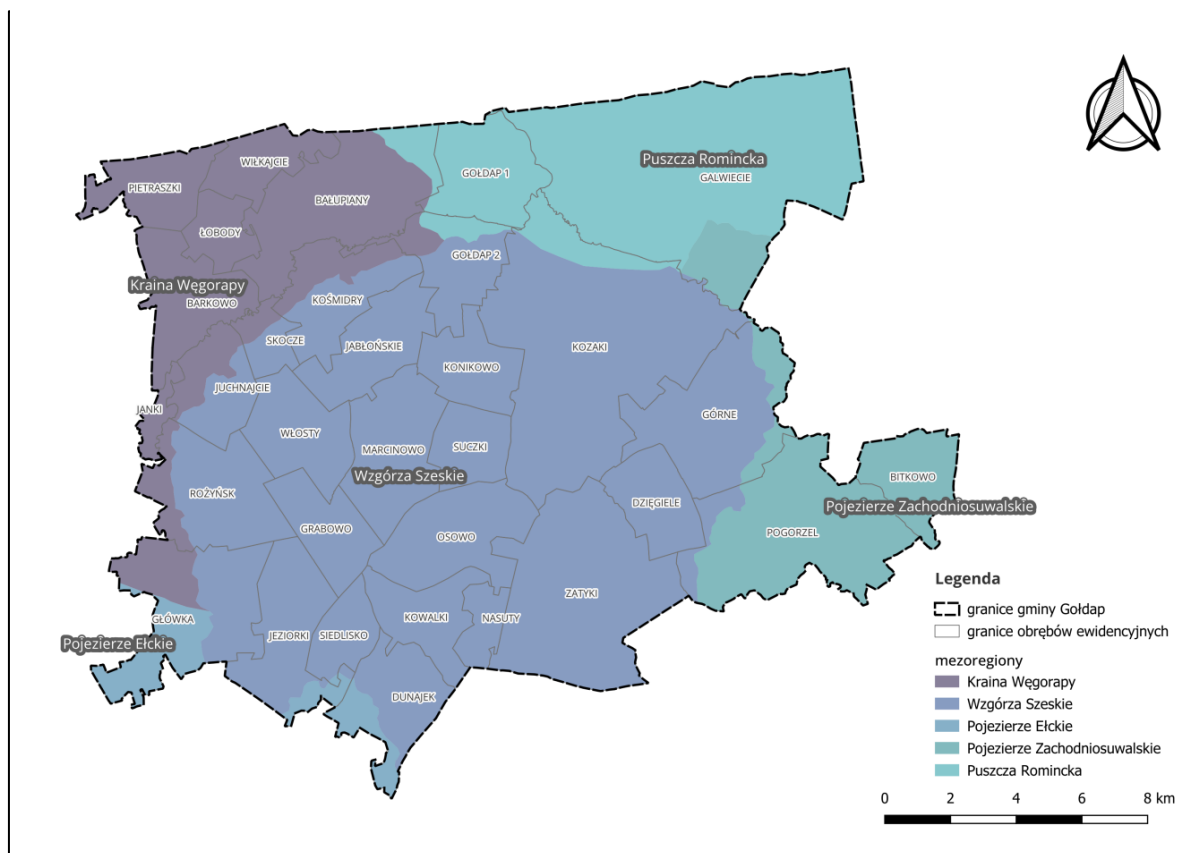
Ryc. 3 Mezoregiony na terenie gminy Gołdap
