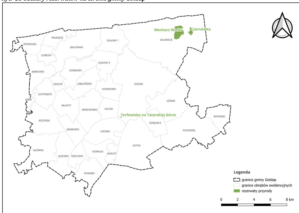
Ryc. 21 Obszary rezerwatów na terenie gminy Gołdap
