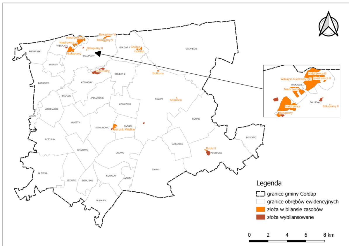
Ryc. 14 Złoża bilansowe i wybilansowane na terenie gminy Gołdap
