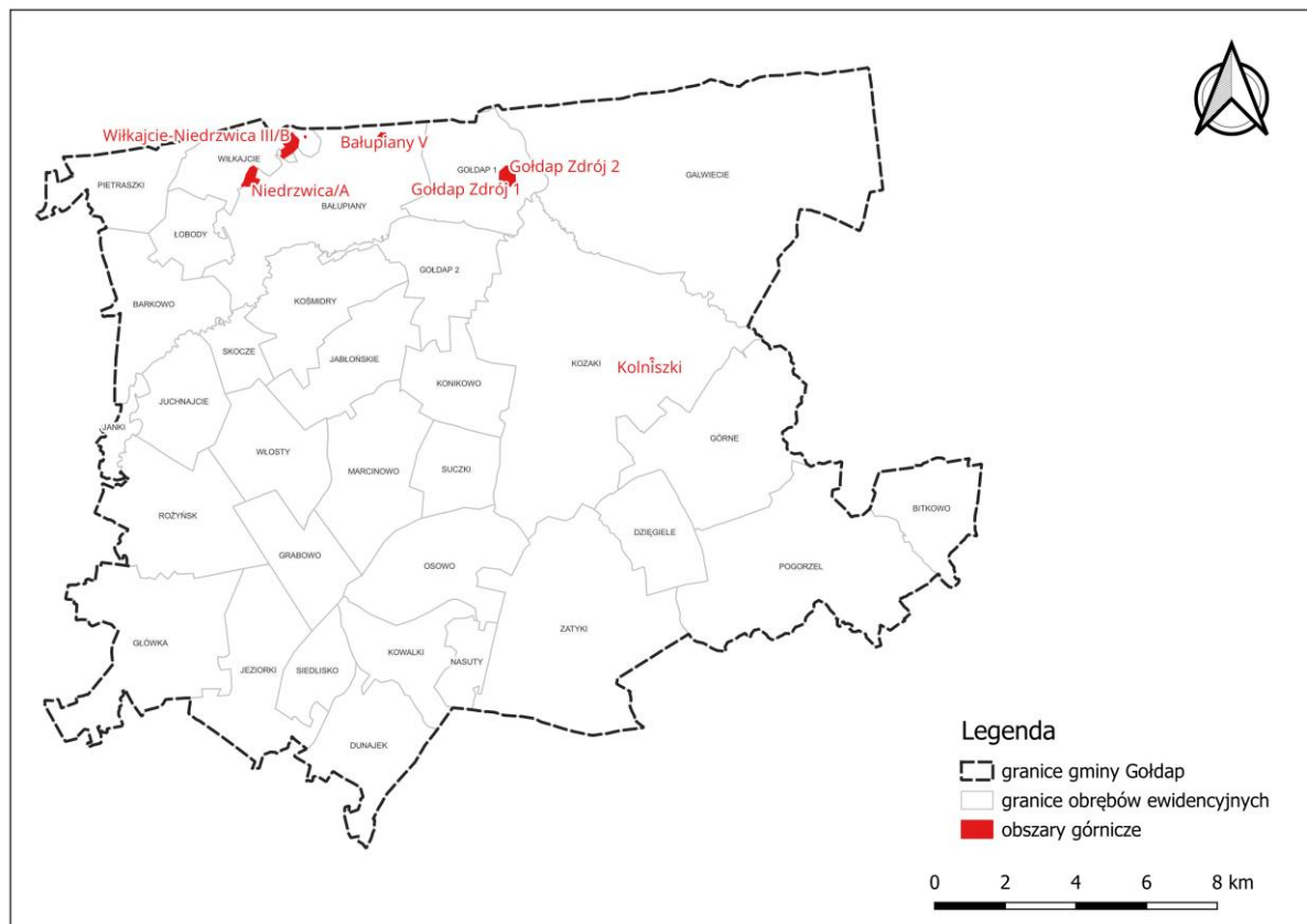
Ryc. 16 Obszary górnicze na terenie gminy Gołdap
