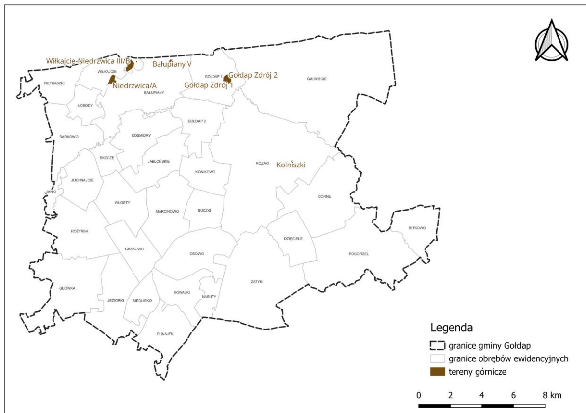
Ryc. 15 Tereny górnicze na terenie gminy Gołdap
