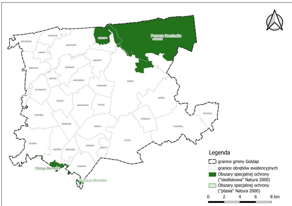
Ryc. 20 Obszary Natura 2000 na terenie gminy Gołdap
