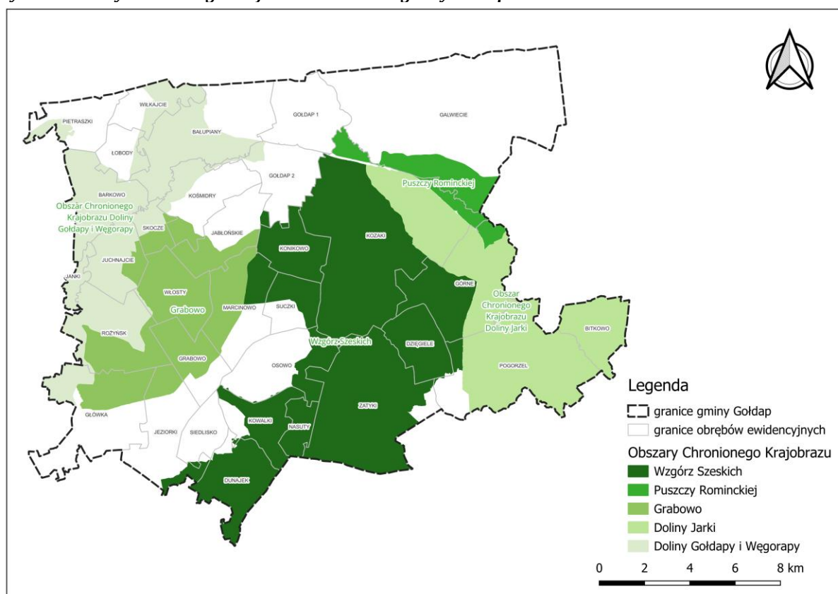
Ryc. 23 Obszary Chronionego Krajobrazu na terenie gminy Gołdap
