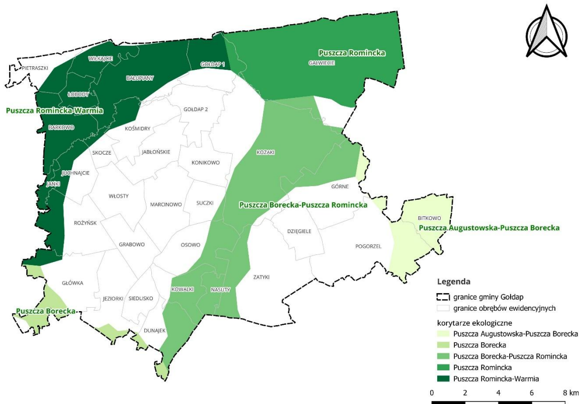
Ryc. 26 Korytarze ekologiczne na terenie gminy Gołdap
