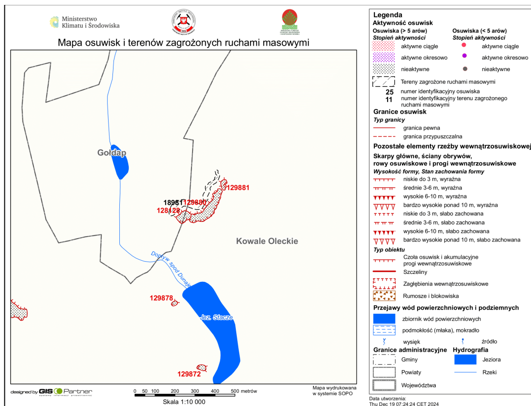
Ryc. 32 Lokalizacja osuwiska i terenów zagrożonych ruchami masowymi w gminie Gołdap
