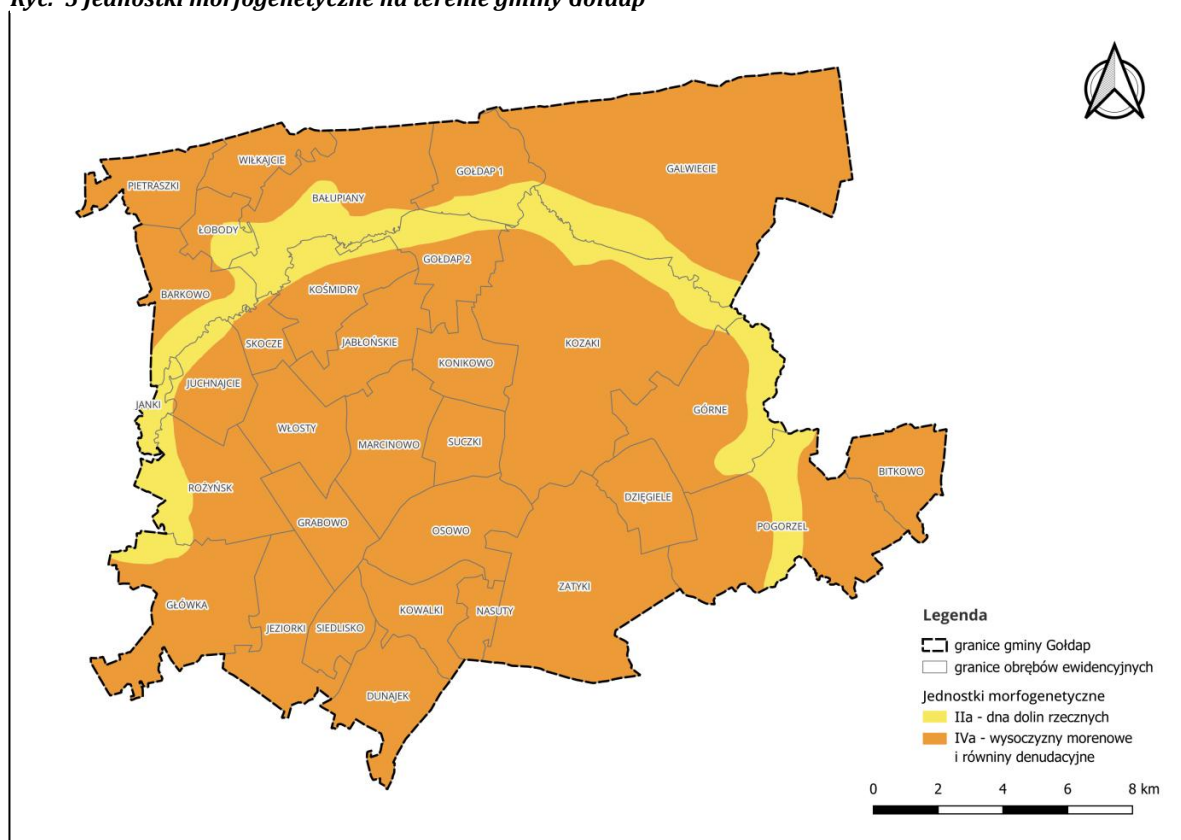
Ryc. 5 Jednostki morfogenetyczne na terenie gminy Gołdap
