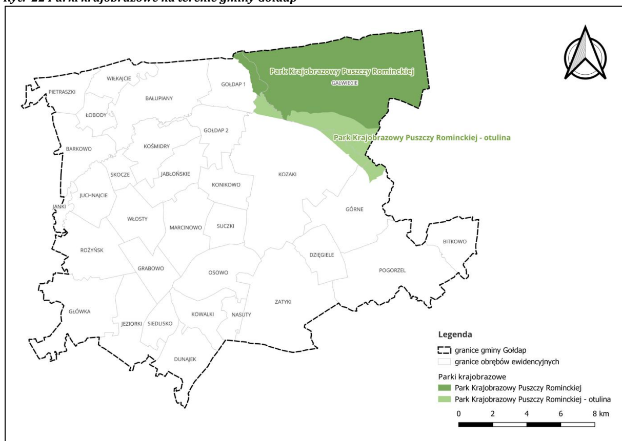
Ryc. 22 Parki krajobrazowe na terenie gminy Gołdap
