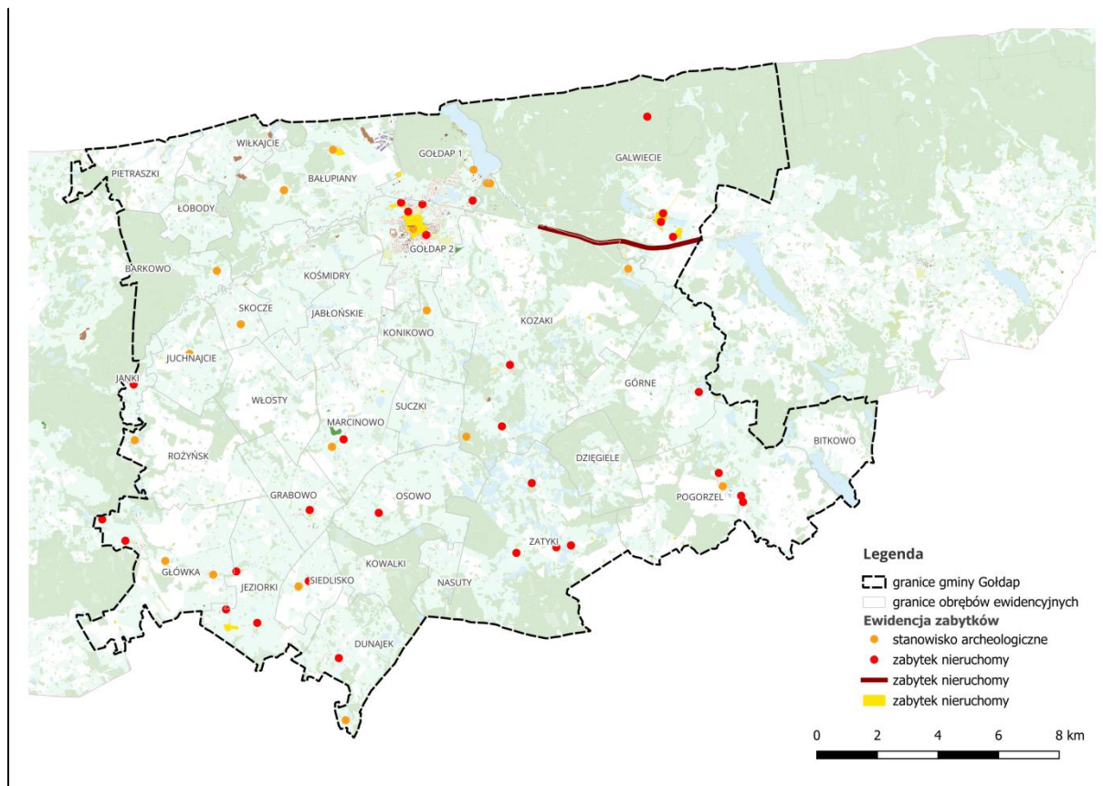
Ryc. 29 Lokalizacja zabytków nieruchomych i stanowisk archeologicznych ujętych w ewidencji zabytków
