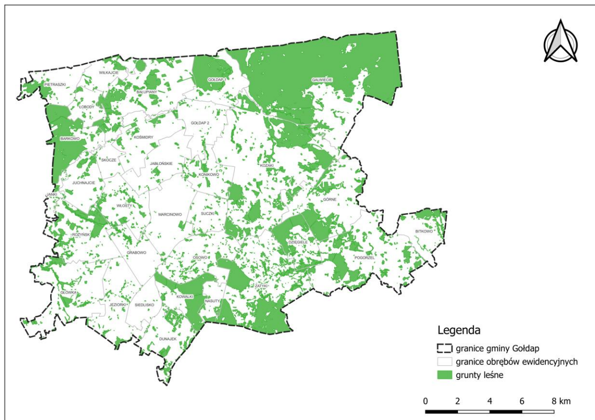
Ryc. 18 Lasy na terenie gminy Gołdap
