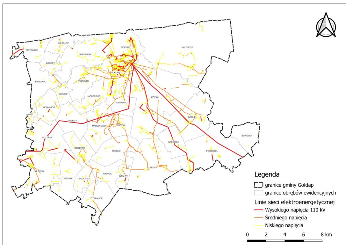
Ryc. 32 Sieć elektroenergetyczna na terenie gminy Gołdap
