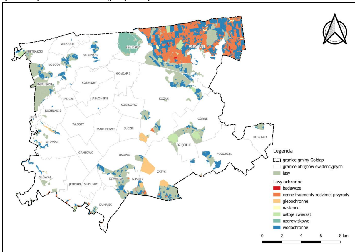
Ryc. 24 Lasy ochronne na terenie gminy Gołdap
