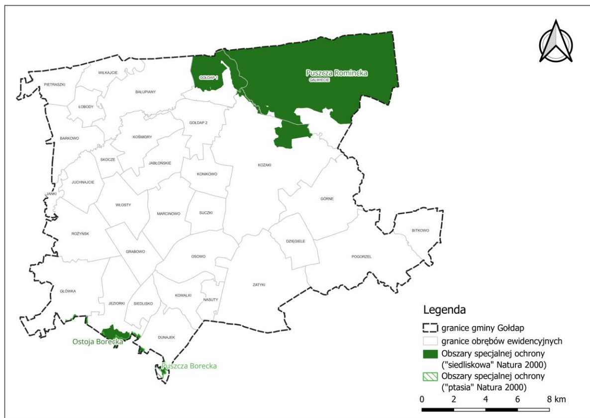
Ryc. 3 Obszary Natura 2000 na terenie gminy Gołdap
