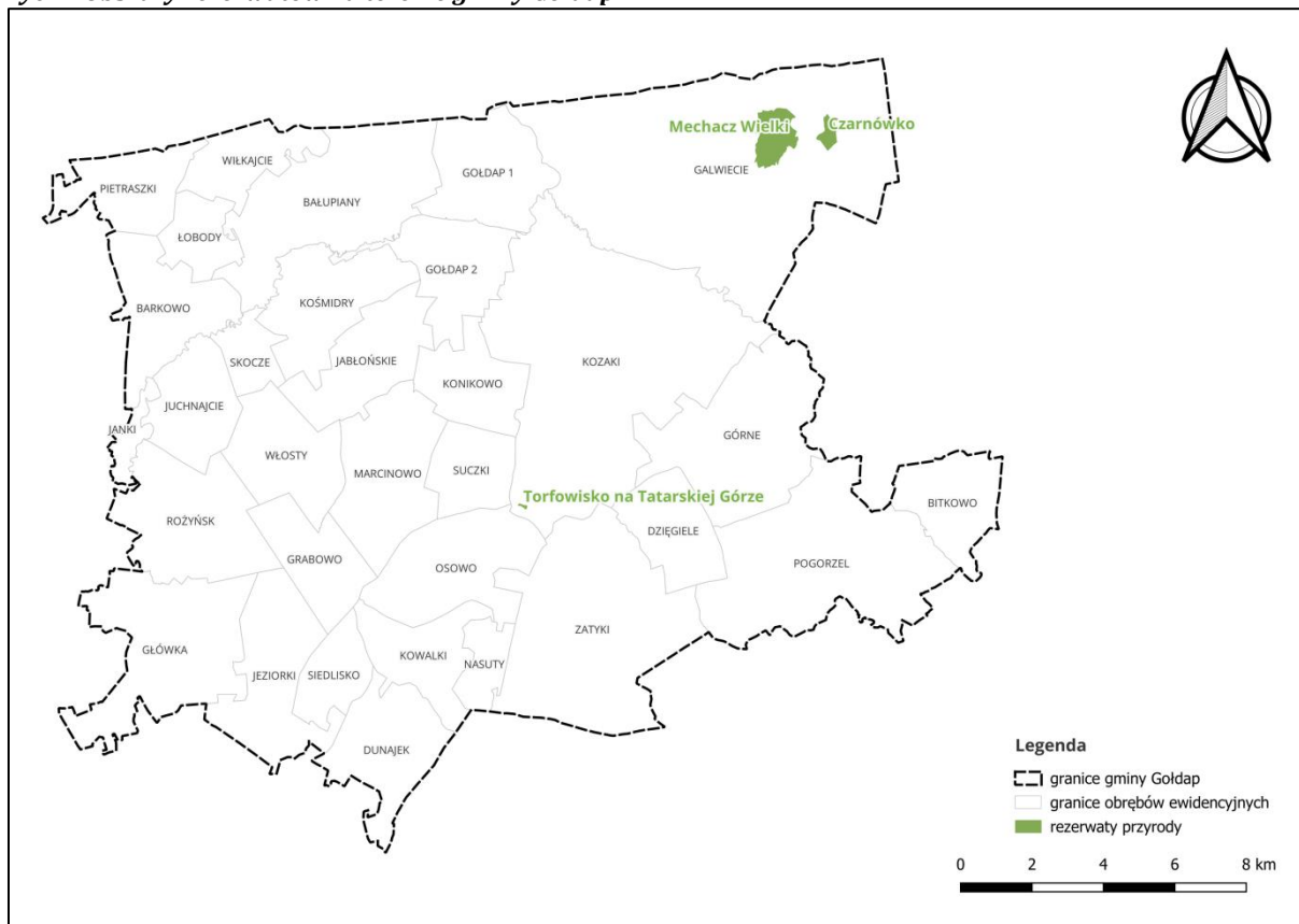
Ryc. 4 Obszary rezerwatów na terenie gminy Gołdap
