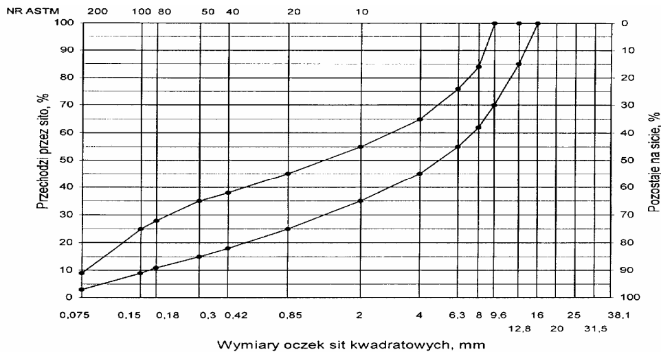
Rys. 6. Krzywe graniczne uziarnienia mieszanki mineralnej BA od 0 do 12,8 mm do warstwy wiążącej, wyrównawczej i wzmocniającej nawierzchni drogi o obciążeniu ruchem KR1 lub KR2.
