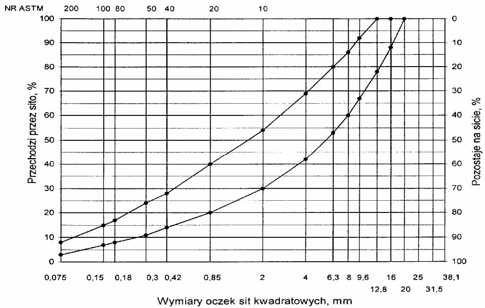
Rys. 5. Krzywe graniczne uziarnienia mieszanki mineralnej BA od 0 do 16 mm do warstwy wiążącej, wyrównawczej i wzmocniającej nawierzchni drogi o obciążeniu ruchem KR1 lub KR2.
