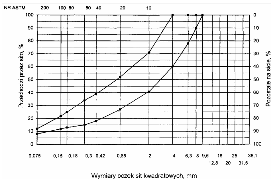
Rys. 3. Krzywe graniczne uziarnienia mieszanki mineralnej BA od 0 do 8mm, od 0 do 6,3 mm do warstwy ścieralnej nawierzchni drogi o obciążeniu ruchem nawierzchni drogi o obciążeniu
