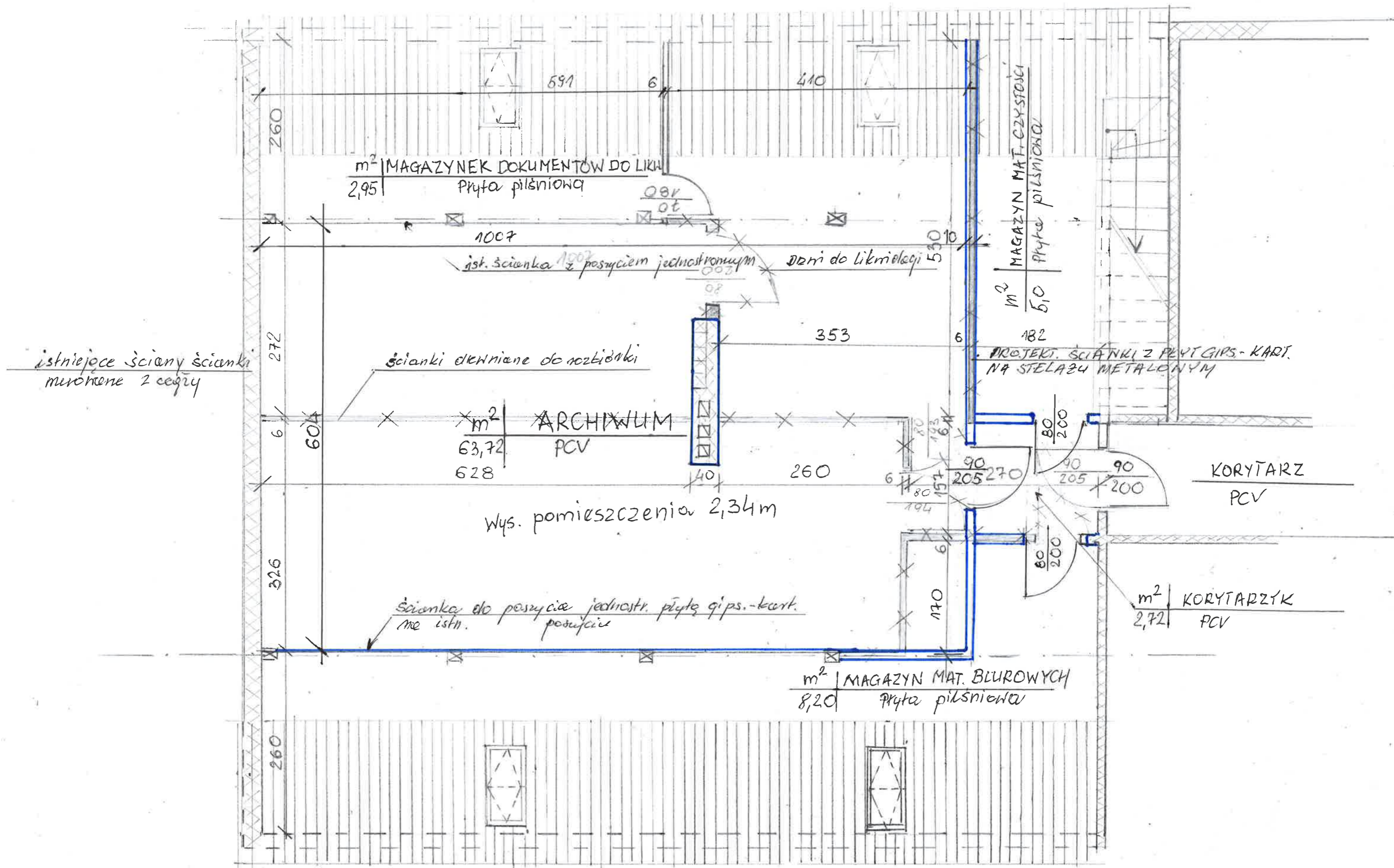
Rzut poziomy 1:50
