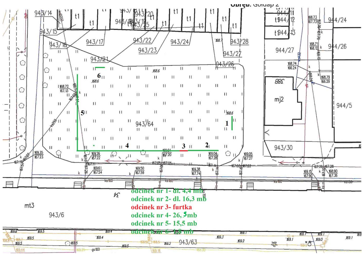
Mapa poglądowa lokalizacji wykonania i rozmieszczenia ogrodzenia
