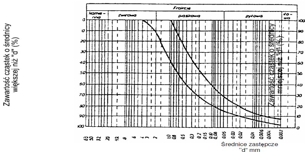
Rysunek 1. Obszar uziarnienia optymalnej mieszanki gliniasto-piaskowej
