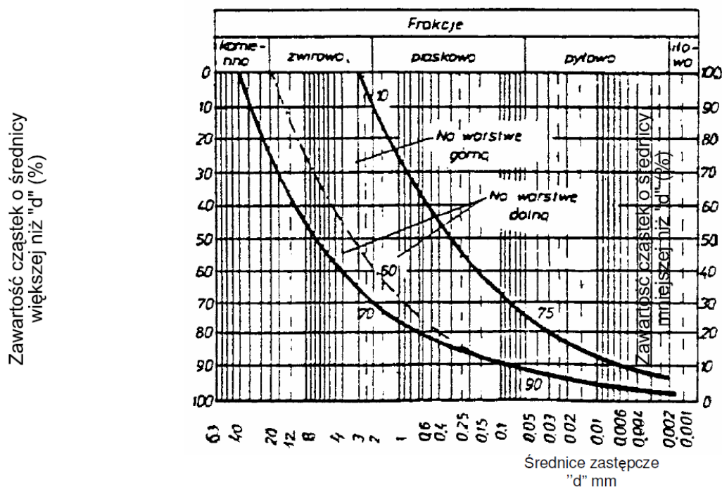
Rysunek 2. Obszar uziarnienia optymalnych mieszanek gliniasto-zwirowych
