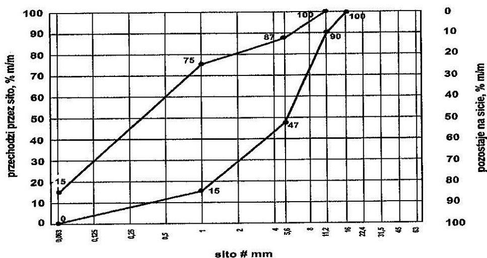
Rys. 2. Krzywe graniczne uziarnienia mieszanki kruszywa 0/11,2 mm do górnej warstwy podłoża ulepszanego
